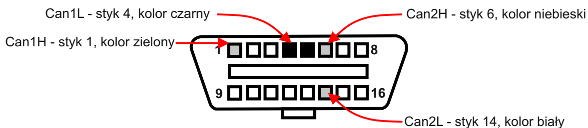
Widok od przodu złącza (czarne styki to dwie masy)
