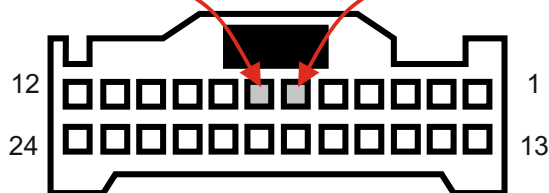
Widok od tyłu złącza (przewodów wchodzących w złącze)
