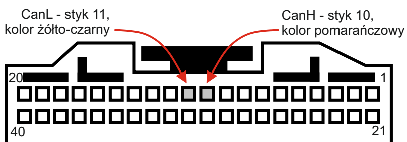
Widok wtyku od strony przewodów
