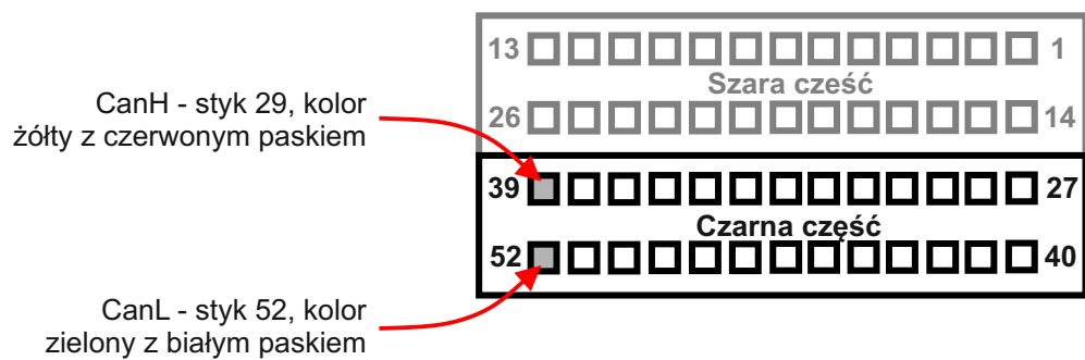
Widok od tyłu wtyku (strony wejścia przewodów)
